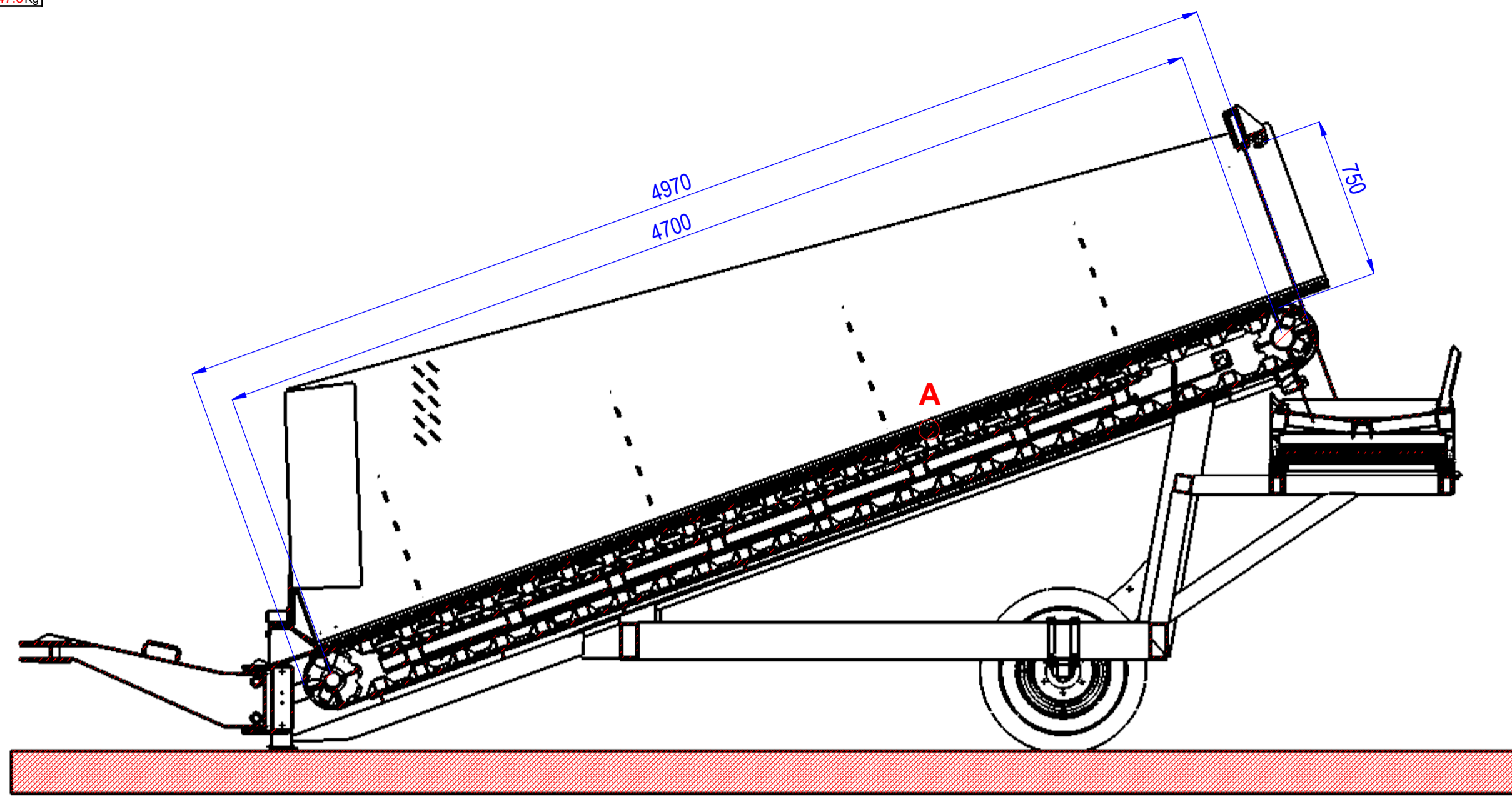
SECTION A-A
